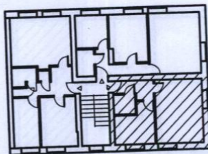
Rzut 1 piętra - klatka C
